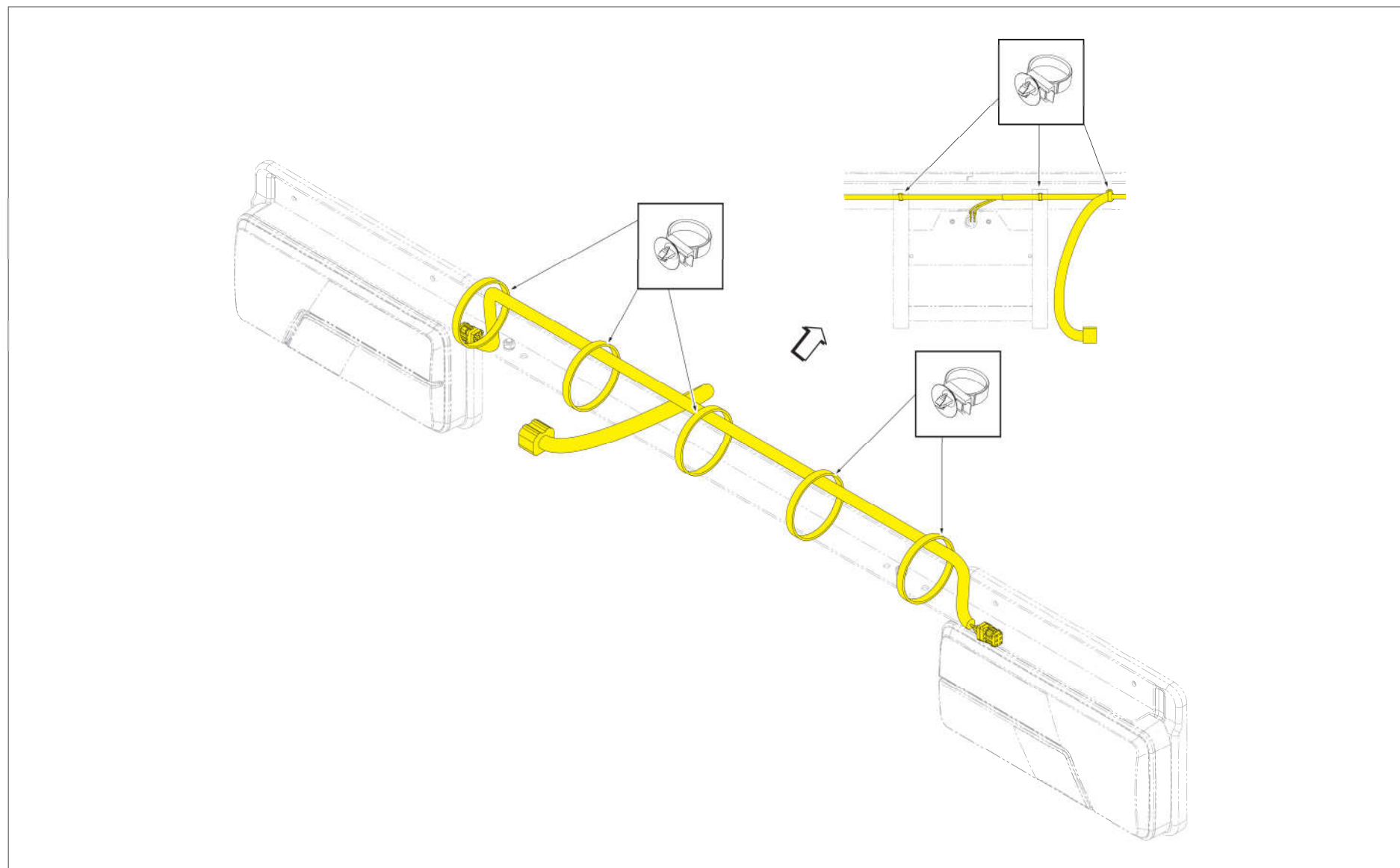
尾灯线束（13A412）安装图
