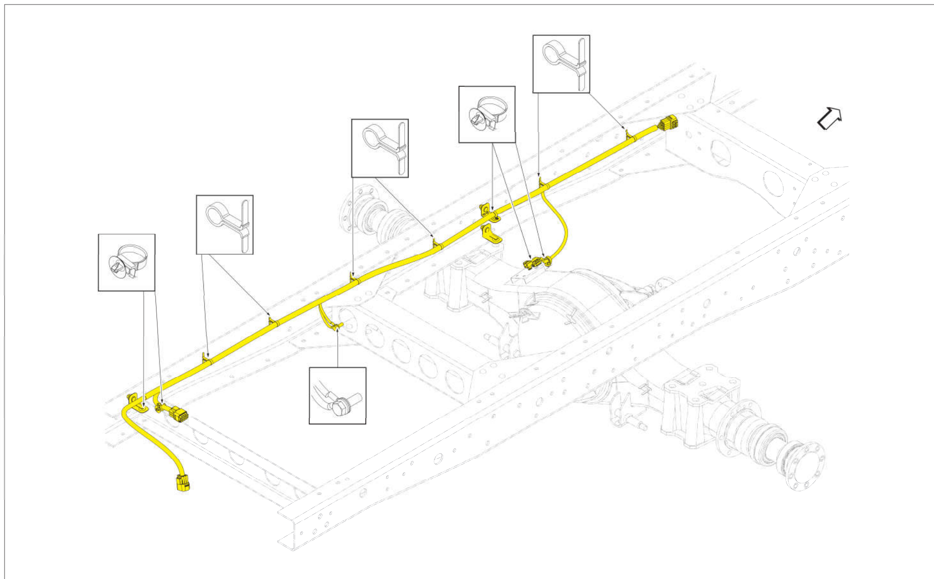
车架后线束 (14034) 安装图
